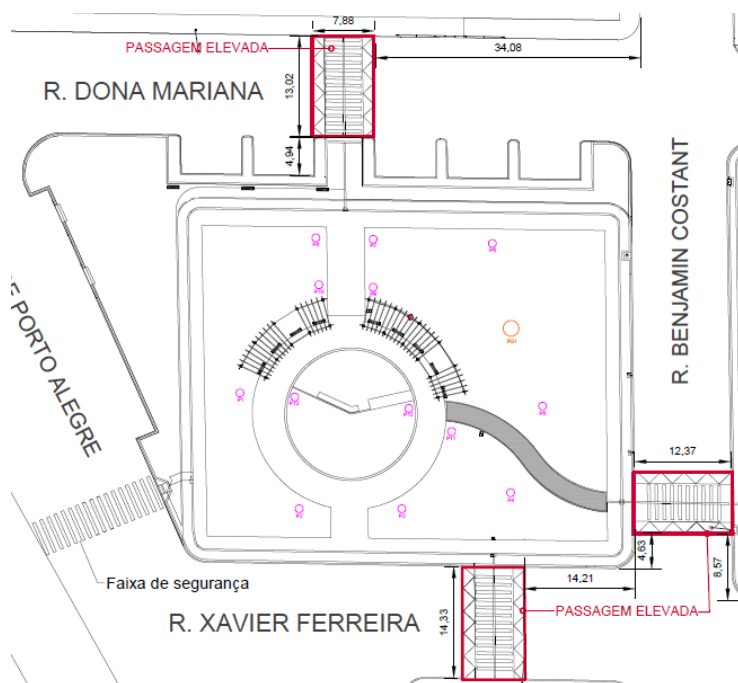
Figura 4 - Plantas de localização dos postes e detalhamento das passagens elevadas e faixa de segurança
